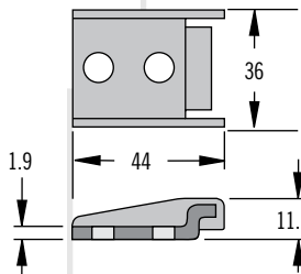
A scomparsa 2 fori
