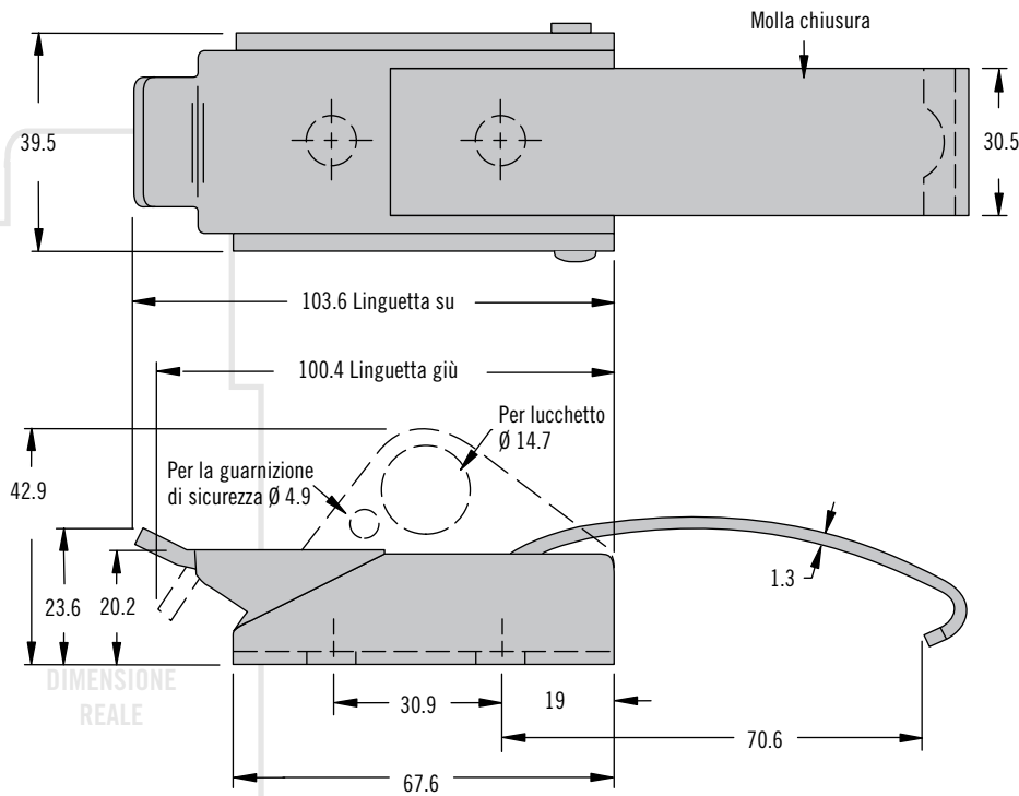
A vista con con montaggio a foro singolo
